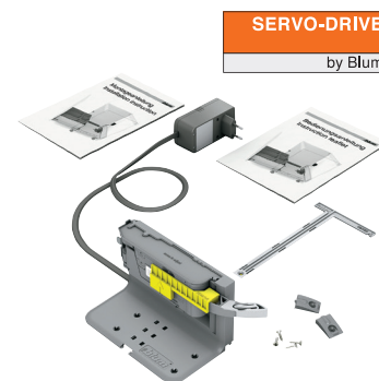
SERVO-DRIVE uno für stehende Müllösungen
